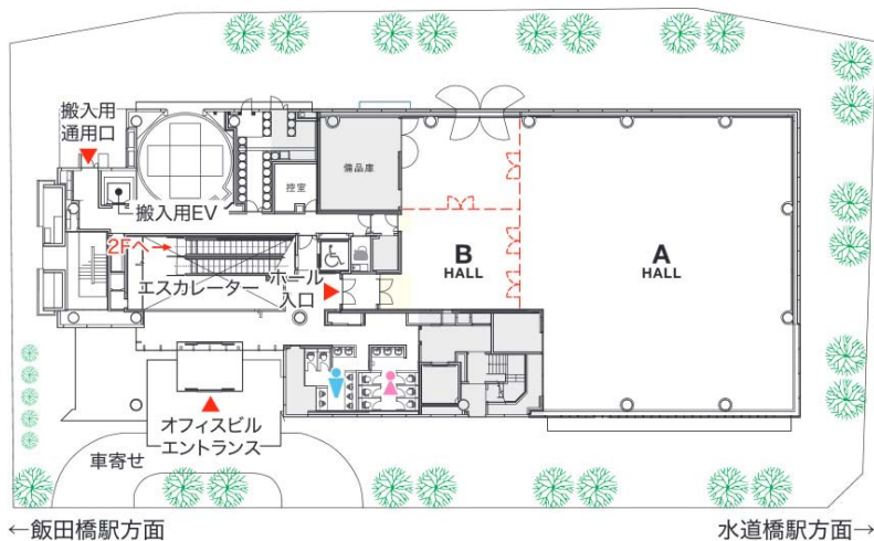
1階平面図
